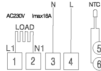
Elekterpõrandaküttega ühendusskeem
