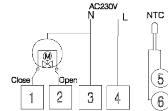
Ajamiga vesipõrandakütte ühendusskeem
